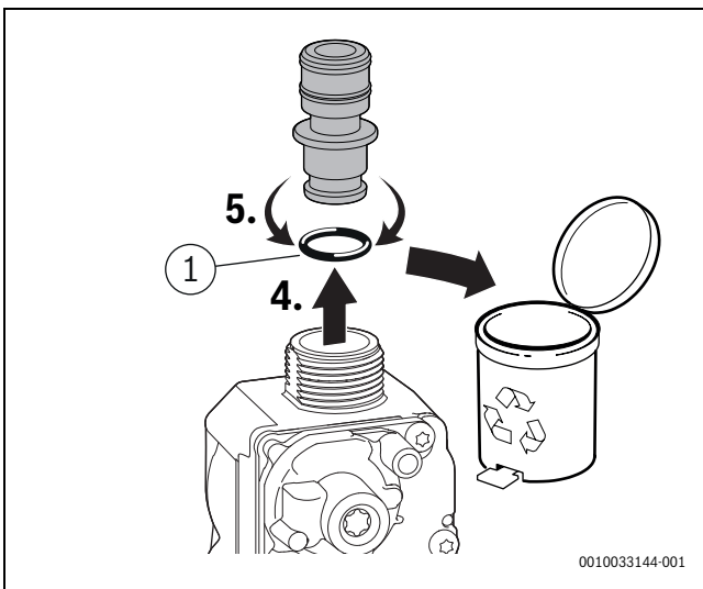
78. ábra A gáz fojtóközdarab levétele
