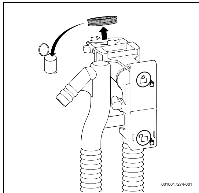
71. ábra A felső tömítés eltávolítása a kondenzvízszifonról
